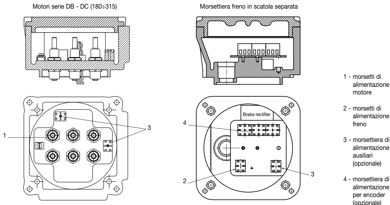
Figura 2T - Scatola morsettiera motori con freno
