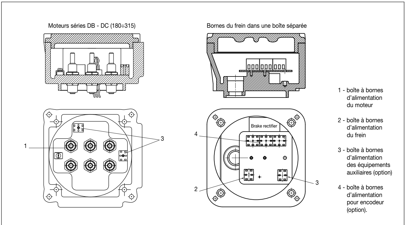
Figure 2T - Boîte à bornes moteurs à frein
