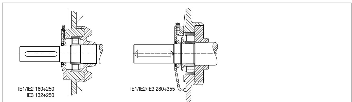
Figure 2I - Roulements à rouleaux - Exécution sur demande DE (avant)
