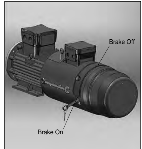
Figura 2G - Desbloqueo manual (opcional bajo pedido) para motores 180÷315 con ventilación asistida
