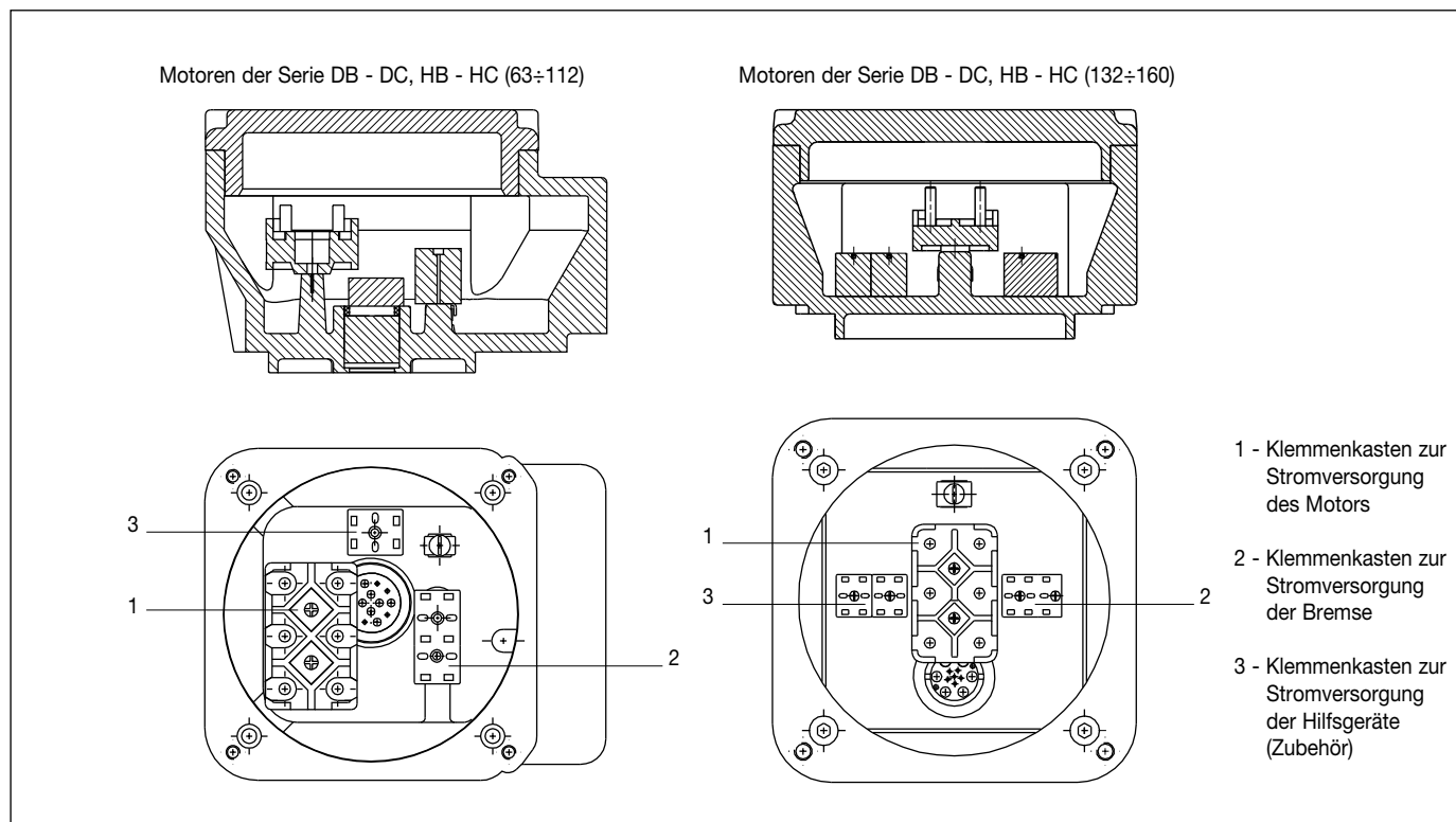
Abbildung 2S - Klemmkasten für Motoren mit Bremse
