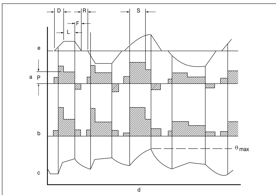
Figura 3L - Régimen S9
