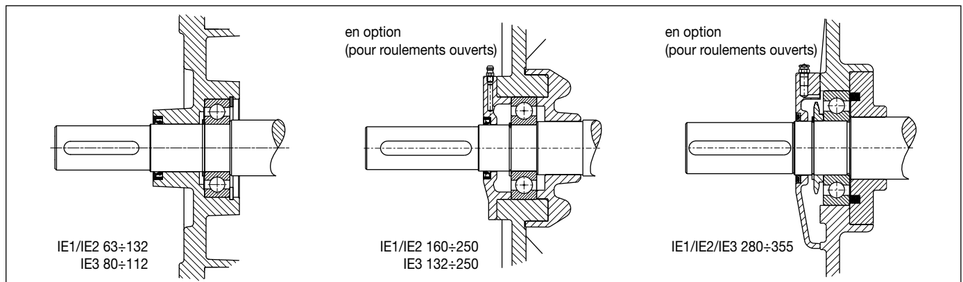
Figure 2H - Roulements à billes - DE (avant)
