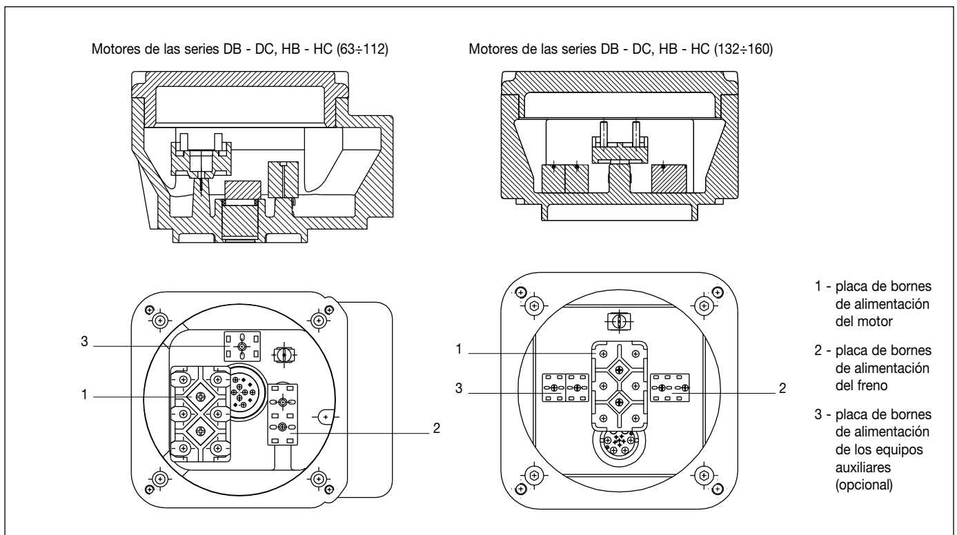
Figura 2S - Caja de conexiones motores con freno
