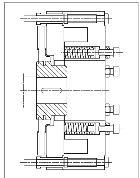
Figura 2D - Esquema de construcción del freno 180÷315
